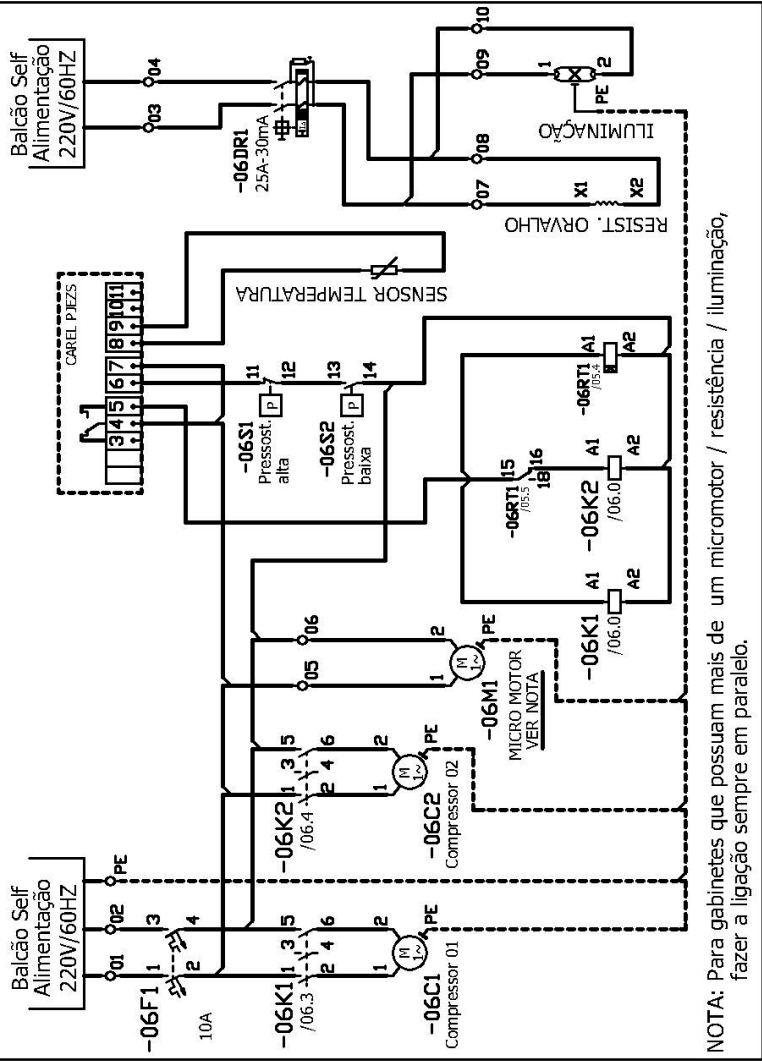
DIAGRAMA ELÉTRICO PLUGIN RESFRIADO – 2COMPRESSORES
